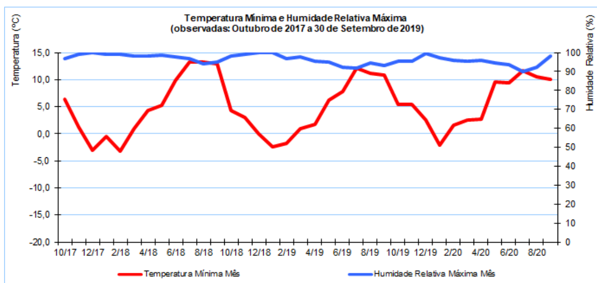
Gráfico XIV – Distribuição da temperatura mínima com a humidade relativa máxima de Outubro/2017 a Setembro/2020. Valores médios mensais
