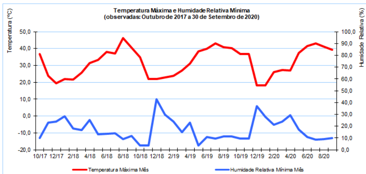
Gráfico XIII – Distribuição da temperatura máxima com a humidade relativa mínima de Outubro/2017 a Setembro/2020. Valores médios mensais
